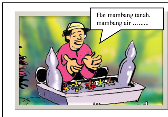
Gambar 2 (Memuja kubur)
